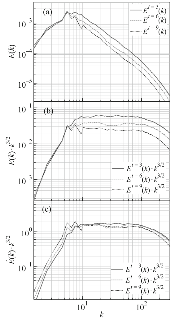
Рис. 1. (Цветной онлайн) (а) – Спектры полной энергии затухающей магнитогидродинамической турбулентности на \beta -плоскости ( \beta = 10 ). (б) – Спектры полной энергии, нормированные на k^{3/2} . (с) – Спектры полной энергии, нормированные на k^{3/2} и скомпенсированные на временную зависимость \sqrt{\epsilon \nu_A} . Сплошными линиями показаны зависимости спектров от волнового числа k для момента времени t = 3 , штрихпунктирными линиями – для момента времени t = 6 , точечными пунктирами – для момента времени t = 9
