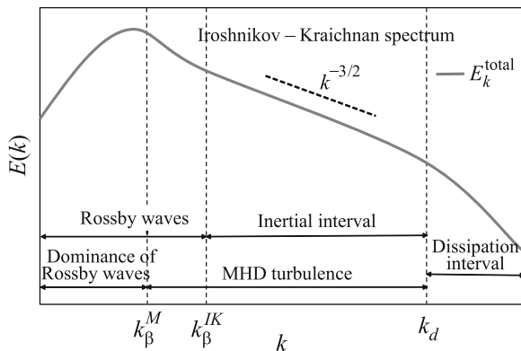
Рис. 3. (Цветной онлайн) Схематическое представление спектра полной энергии двумерной затухающей МГД турбулентности на \beta -плоскости.
