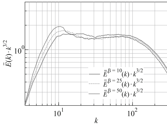
Рис. 2. (Цветной онлайн) Спектры полной энергии, нормированные на k^{3/2} , скомпенсированные на временную зависимость \sqrt{\epsilon v_A} и усредненные на временном промежутке t = 3 - 6 для различных параметров Россби. Сплошной линией показана зависимость модифицированного спектра для параметра Россби \beta = 10 от волнового числа k , штрихпунктирной линией – для параметра Россби \beta = 25 , точечным пунктиром – для параметра Россби \beta = 50
