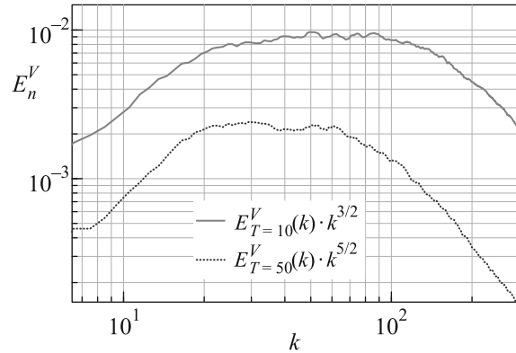
Рис. 5. (Цветной онлайн) Нормированные спектры кинетической энергии затухающей магнитогидродинамической турбулентности на \beta -плоскости ( \beta = 10 ) для моментов времени t = 10; 50
