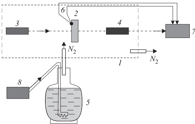
Рис. 1. (Цветной онлайн) Схема установки для изучения пропускания тонкой пленки льда 0; конденсированной на прозрачную диэлектрическую пластину: 1 – холодильная камера; 2 – диэлектрическая подложка с осажденным из газовой фазы льдом 0; 3 – лазер; 4 – фотодетектор с усилителем; 5 – сосуд Дьюара с жидким азотом и резистором-испарителем; 6 – термопара; 7 – система сбора информации; 8 – стабилизированный источник тока для питания испарителя
