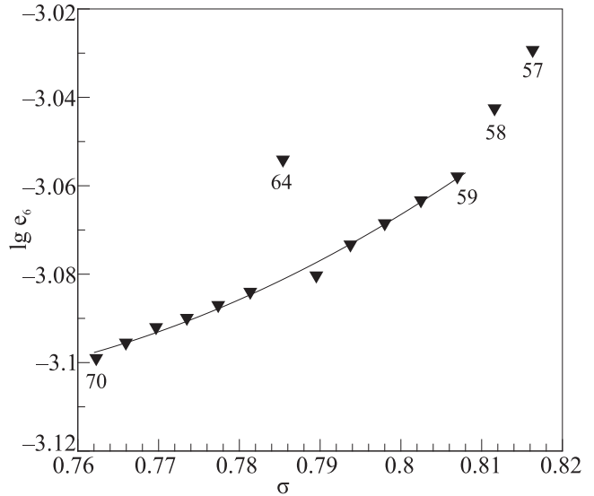
Рис. 3. Зависимость \lg e_6(\sigma) , построенная по экспериментальным потенциалам ионизации \text{IP}_1 из базы [1] для лантанидов, в которых ионизируется 6s-электрон. Линия – квадратичная аппроксимация (4)
