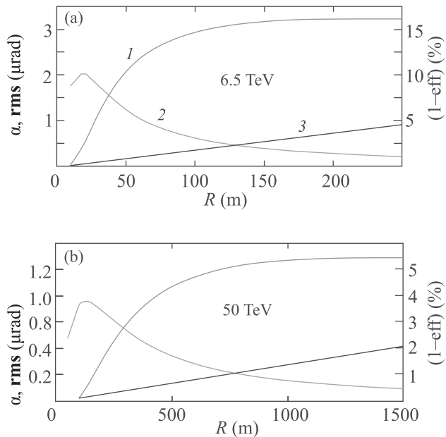
Рис. 2. (Цветной онлайн) Зависимость параметров отражения от радиуса изгиба кристалла: 1 – средний угол отражения \alpha , 2 – среднеквадратичное значение углового распределения \text{rms} ; 3 – величина (1 - \text{eff})
