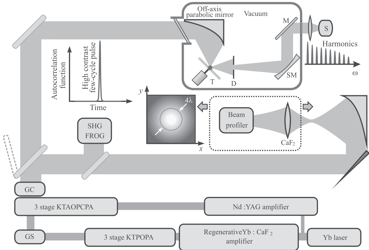
Рис. 1. (Цветной онлайн) Экспериментальная схема: ОРА – оптический параметрический усилитель, ОРСПА – оптический параметрический усилитель chirпированных импульсов, GS – решеточно-призмный стретчер, GC – решеточный компрессор, T – мишень, M – зеркало, D – диафрагма, S – спектрометр
