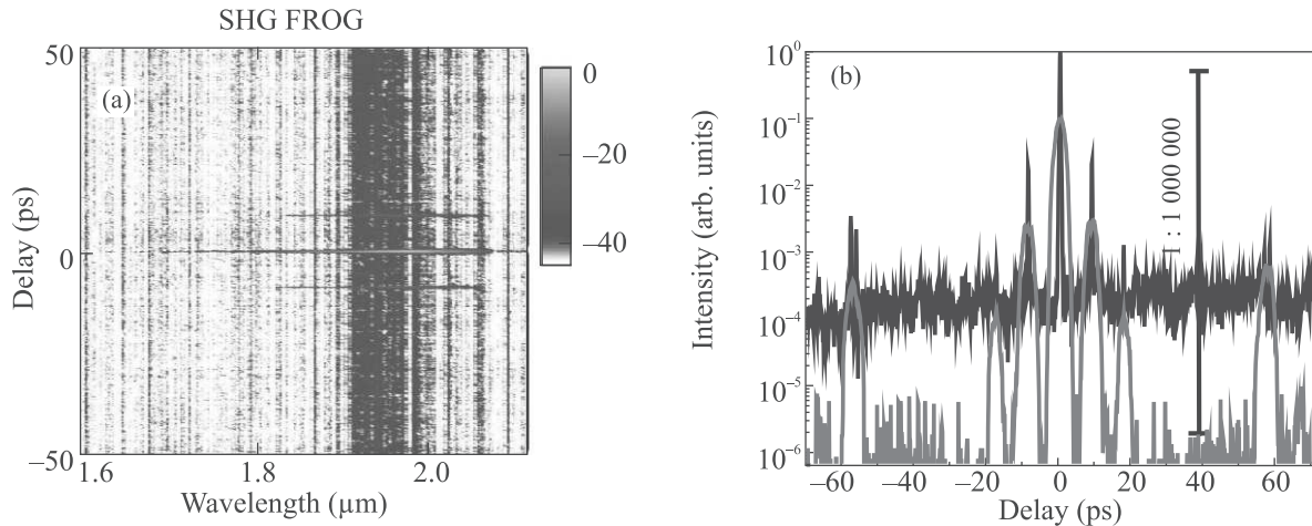
Рис. 4. (Цветной онлайн) Характерная SHG-FROG-спектрограмма (а) и полученная на основе обработки этой спектрограммы автокорреляционная функция интенсивности (б) импульса среднего ИК-излучения. Розовой кривой показана АК-функция интенсивности импульса среднего ИК-излучения с наложенным с помощью решеточного компрессора профилем фазы, соответствующим параметру чирпа 0.05 \text{ ps}^2
