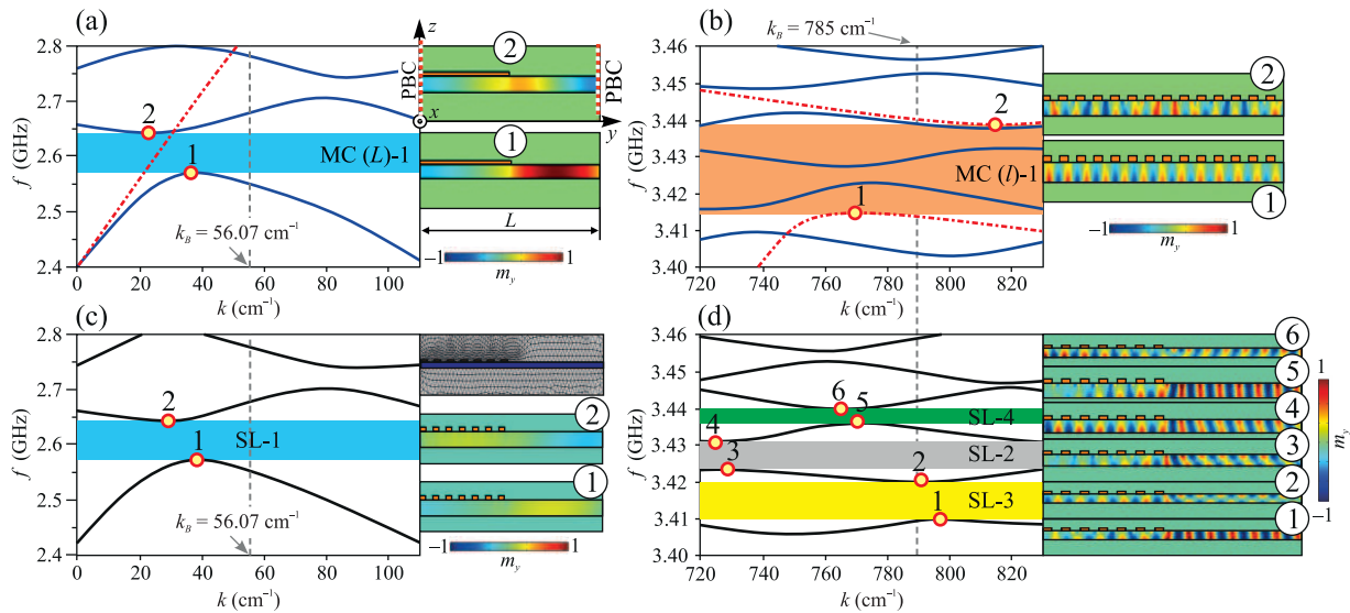
Рис. 3. (Цветной онлайн) Дисперсионные характеристики ПМСВ (а), (b) в МК с периодом l (красные кривые), МК с периодом L (синие кривые), (c), (d) – в МК с двумя периодами (черные кривые). Закрашенные области соответствуют запрещенным зонам. На правых панелях приведено распределение m_y компоненты намагниченности для частот, соответствующих краям ЗЗ. На правой панели к рис. (c) показан фрагмент разбиения расчетной области на элементы для примитивной ячейки магнной суперрешетки. Расчетные параметры: \epsilon = 14 , N = 14 , d_1 = 3 мкм, остальные параметры как на рис. 2
