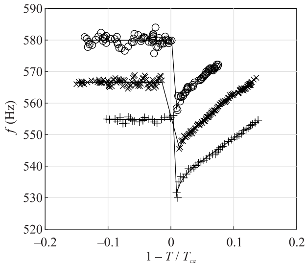
Рис. 2. Кружки, кресты, плюсы – зависимость от температуры частоты механической колебательной моды, наблюдаемой в эксперименте [12], для давлений 7.1, 15.6, 29.3 бар соответственно. Сплошные линии – подгонка теоретическими зависимостями (17), (18), в которых использовались выражения (16), (19). Зависимость \rho_s^\pm(T) взята из (20), где использовались значения коэффициентов \beta_i чистого ^3\text{He} . Подгонка произведена для случая, когда снаружи аэрогеля существует А-фаза
