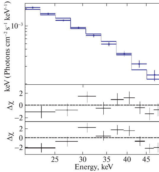
Рис. 3. Вверху: энергетический спектр излучения от скопления Змееносец по данным телескопа IBIS в диапазоне энергий 20–50 кэВ с ошибками (синие бины) и тепловая модель APEC спектра (синяя линия). Внизу: невязки \{\Delta\chi = (\text{data} - \text{model})/\text{error}\} тепловой (APEC; сверху) и степенной (powerlaw; снизу) моделей спектра.
