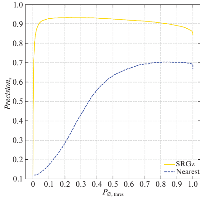
Рис. 11. Зависимость P_{0,thres} — полная точность оптического отождествления рентгеновских источников ePOZITA. Сплошной линией показана лучшая модель отождествления SRGz, штриховой — модель отождествления по ближайшему оптическому соседу. Максимальная точность отождествления в модели SRGz составляет Precision_{X,max} = 0.93 (соответствует P_{0,thres} = 0.24 ).
