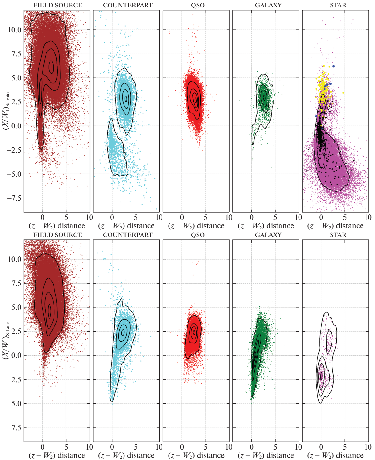
Рис. 8. Разграничение оптических компаньонов точечных рентгеновских источников двухлетнего обзора eРОЗИТА для спектральных/астрометрических классов на плоскости цветовой расстояние (z - W_2) — отношение рентген/ИК (X/W_1)_{\text{Salvato}} (подробности по обозначениям и графикам см. текст и подпись к рис. 5).
