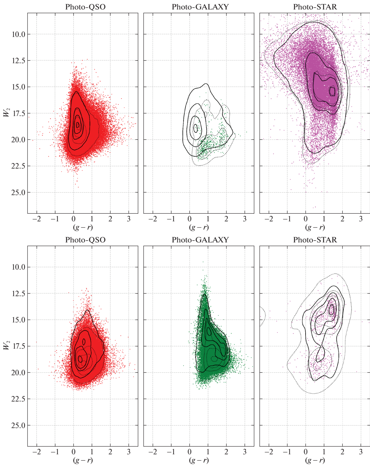
Рис. 21. Фотометрическая классификация SRGz оптических компаньонов точечных рентгеновских источников двухлетнего обзора eROZITA на плоскости (g-r) — величина W_2 (подробнее см. подпись к рис. 20).
