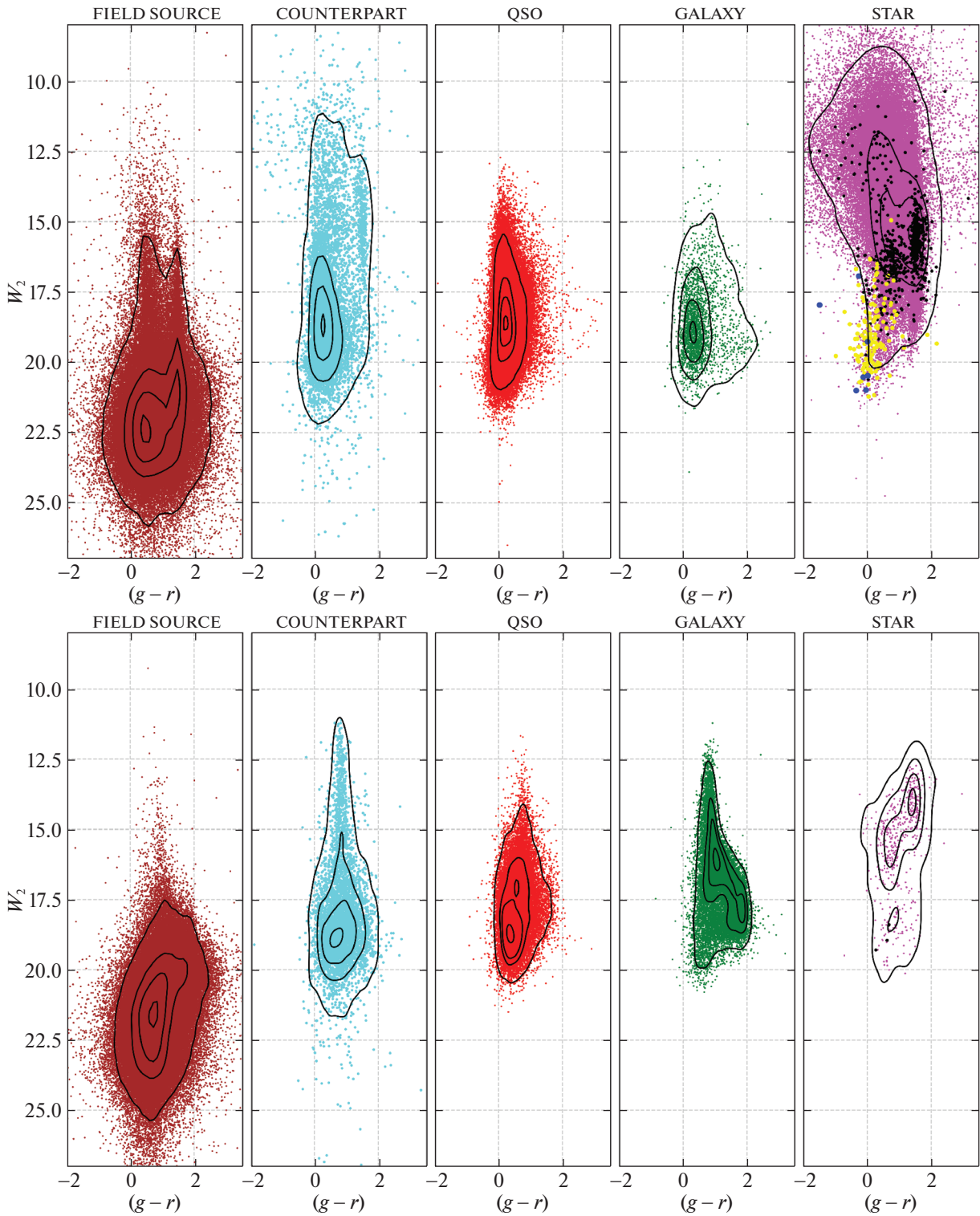
Рис. 6. Разграничение оптических компаньонов точечных рентгеновских источников двухлетнего обзора eROSITA для спектральных/астрометрических классов на плоскости цвет (g-r) — величина W_2 (подробности по обозначениям и графикам см. текст и подпись к рис. 5).
