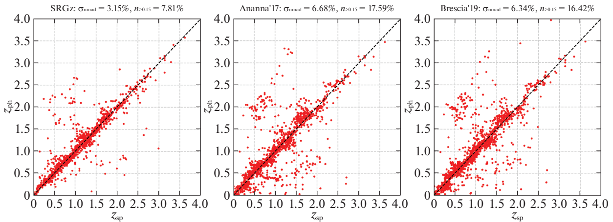
Рис. 24. Точность фотометрических красных смещений оптических компаньонов точечных рентгеновских источников ePOZITA в области Stripe82X разными методами: слева — SRGz, в центре — Ананна и др. (2017), справа — Брешиа и др. (2019).
