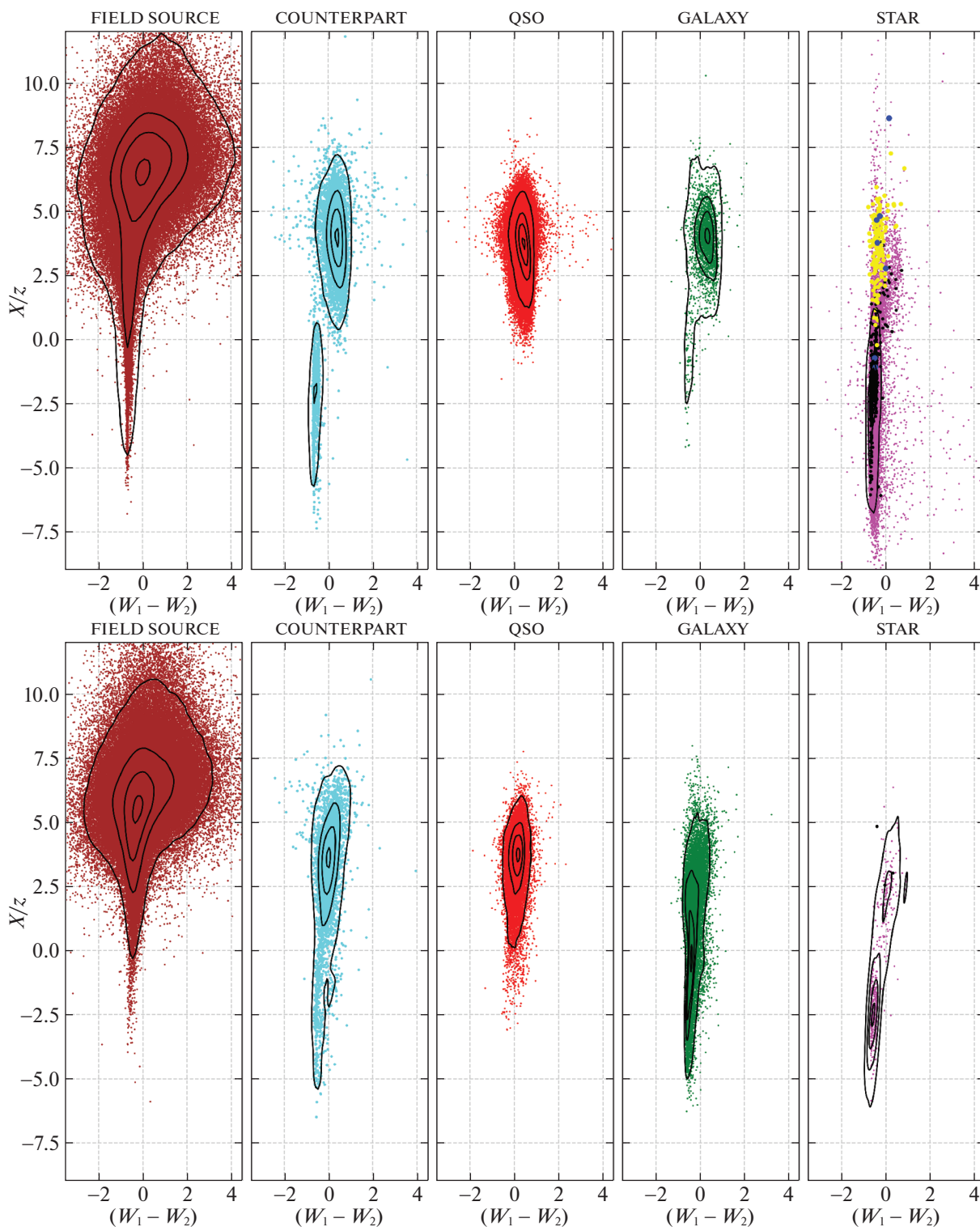
Рис. 7. Разграничение оптических компаньонов точечных рентгеновских источников двухлетнего обзора eROSITA для спектральных/астрометрических классов на плоскости цвет (W_1 - W_2) — отношение рентген/оптика X/z (подробности по обозначениям и графикам см. текст и подпись к рис. 5).
