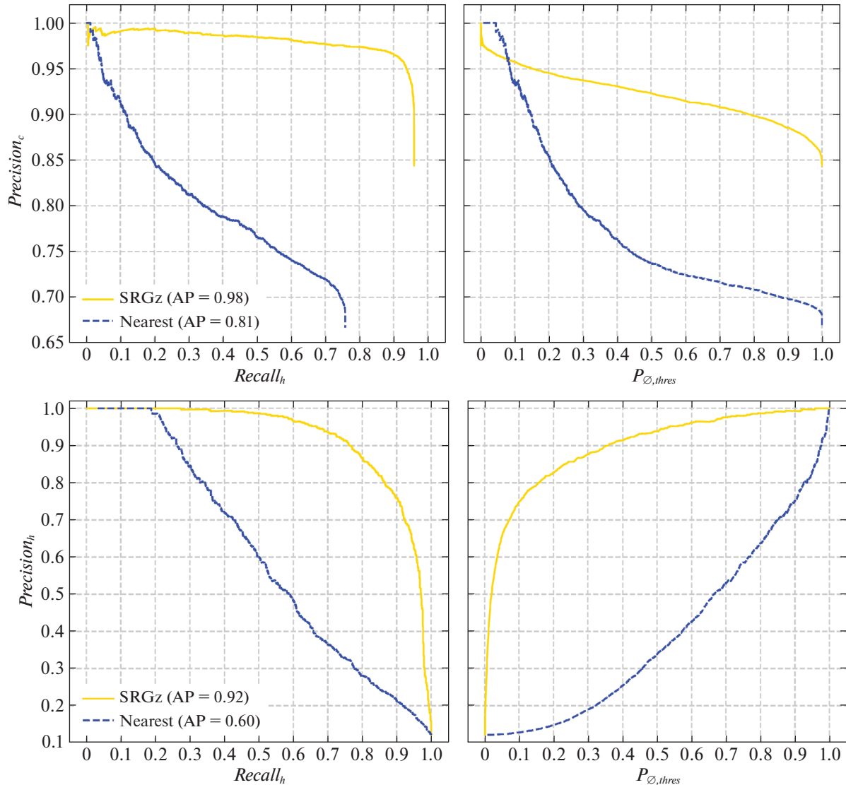
Рис. 10. Зависимости точность — полнота (слева) и P_{\emptyset,thres} — полнота (справа) отождествления оптических компаньонов (верхняя панель) и “бездомных” в DESI LIS (нижняя панель) рентгеновских объектов на тестовой выборке. Сплошными линиями показана лучшая модель отождествления SRGz, штриховыми — модель отождествления по ближайшему оптическому соседу. Максимальная полнота отождествления оптических компаньонов рентгеновских источников ePOZITA для представленной модели SRGz составляет Recall_{c,max} \approx 96\% .
