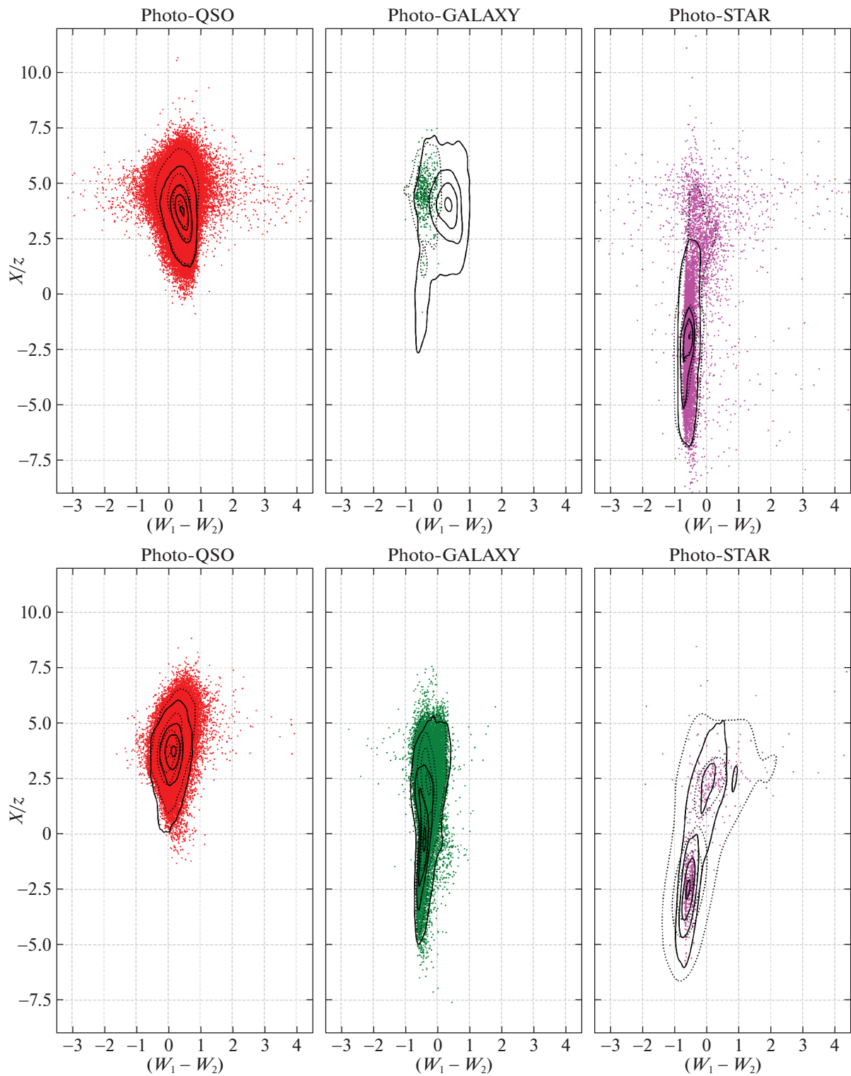
Рис. 22. Фотометрическая классификация SRGz оптических компаньонов точечных рентгеновских источников двух-летнего обзора eROZITA на плоскости цвет (W_1 - W_2) — отношение рентген/оптика X/z (подробнее см. подпись к рис. 20).
