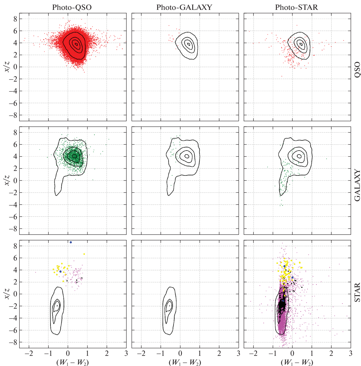
Рис. 14. Фотометрическая классификация SRGz точечных оптических объектов ( type = PSF, DUP ) обзора DESI LIS, являющихся компаньонами точечных рентгеновских источников двухлетнего обзора ePOZITA (в тестовой области SDSS), на плоскости цвет (W_1 - W_2) — отношение рентген/оптика X/z (подробное описание см. рис. 12).
