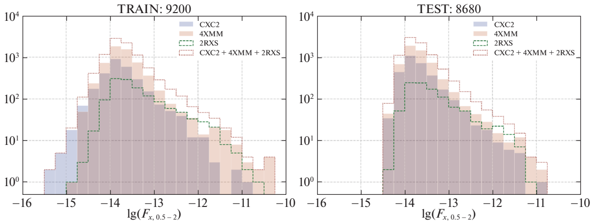
Рис. 4. Распределение по рентгеновому потоку источников eРОЗИТА из тренировочной (левая панель) и тестовой (правая панель) выборок с оптическими компаньонами найденных из пересечения с рентгеновскими обзорами CXC2, 4XMM, 2RXS. Показаны распределение для всех источников и для выборок объектов из каждого вспомогательного рентгеновского обзор по отдельности.
