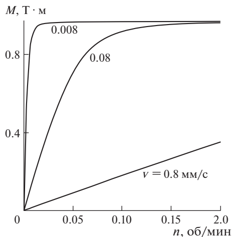
Рис. 3. Влияние скорости кручения на крутящий момент при осадке для значений линейной скорости v : 0.008 мм/с; 0.08 мм/с; 0.8 мм/с при коэффициенте \psi = 0.2 .
