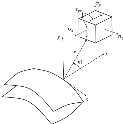
Рис. 1. Напряженное состояние по фронту трещины нормального отрыва.
