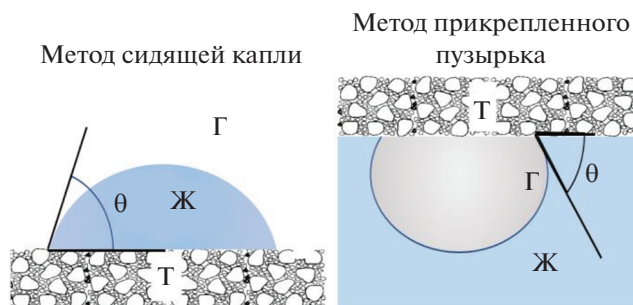
Рис. 1. Схемы измерения контактного угла смачивания \theta в методе сидящей капли и прикрепленного пузырька: Т — твердая поверхность, Ж — жидкая фаза (вода), Г — газовая фаза (воздух).
