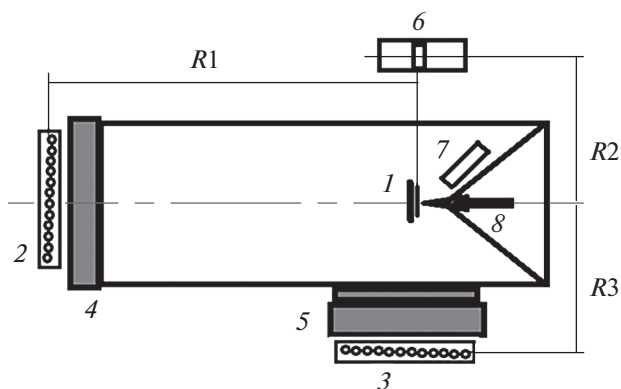
Рис. 1. Схема эксперимента: 1 – мишень на держателе, охлаждаемом водой; 2 и 3 – нейтронные детекторы на основе ^{12}\text{C} -счетчиков, 4 и 5 – радиаторы из оргстекла толщиной 7 и 10 см соответственно; 6 – сцинтилляционный детектор нейтронов; 7 – алмазный детектор заряженных частиц; 8 – ионный пучок. Расстояния от мишени до детекторов R_1 = 100 , R_2 = 45 , R_3 = 40 см.
