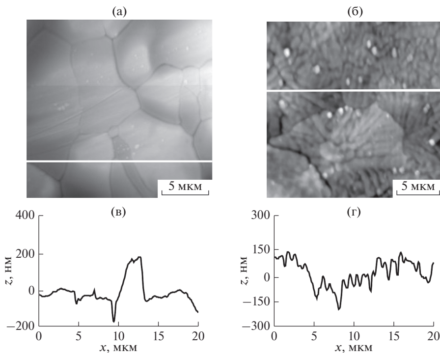
Рис. 1. АСМ-изображения поверхностей A (а) и B (б) свежезакаленных фольг сплава 1421 и соответствующие диаграммы распределения неровностей (в) и (г) вдоль линий сканирования, выделенных на (а) и (б).
