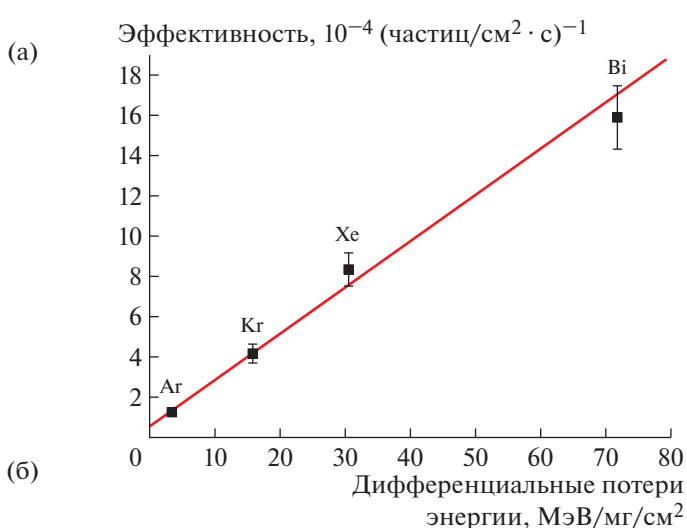
Рис. 3. Зависимость эффективности недеградирующего многоканального детектора от дифференциальных потерь энергии регистрируемых тяжелых ионов в нержавеющей стали.
