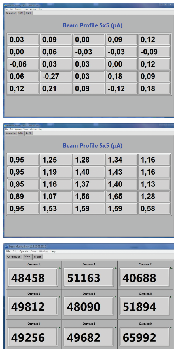
Рис. 2. Изображения с экрана внешнего управляющего компьютера при измерении с помощью токового многоканального профилометра: а — в отсутствие пучка, б — с пучком ионов ^{84}\text{Kr} с энергией 22.9 МэВ/нуклон, плотностью потока 5 \cdot 10^4 ионов/см ^2 ; в — при измерении этого пучка с помощью 9-канального сцинтилляционного профилометра.
