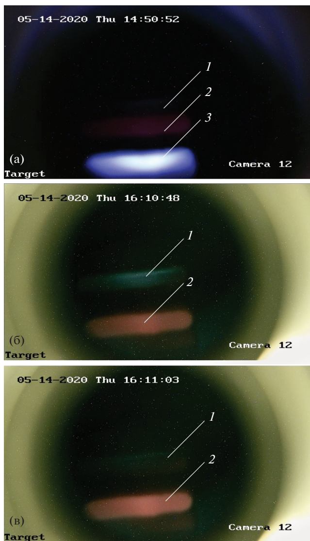
Рис. 5. Свечение, регистрируемое видеокамерой Hikvision при облучении литиевой мишени компонентами пучка заряженных частиц, при токе поворотного магнита 14 А (а), 68 А (б) и 68 А и увеличенном в 2 раза газонапуске в обдирочную мишень (в). 1 – свечение, вызванное нейтралами (атомами водорода), 2 – ионами аргона, 3 – протонами.
