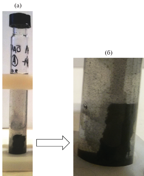
Рис. 1. Брусек стальной арматуры в питательной среде Видделя, инокулированной Desulfovibrio sp., на 14 сут культивирования (а, б — при увеличении, виден черный осадок нерастворимого в воде сульфида железа FeS).
