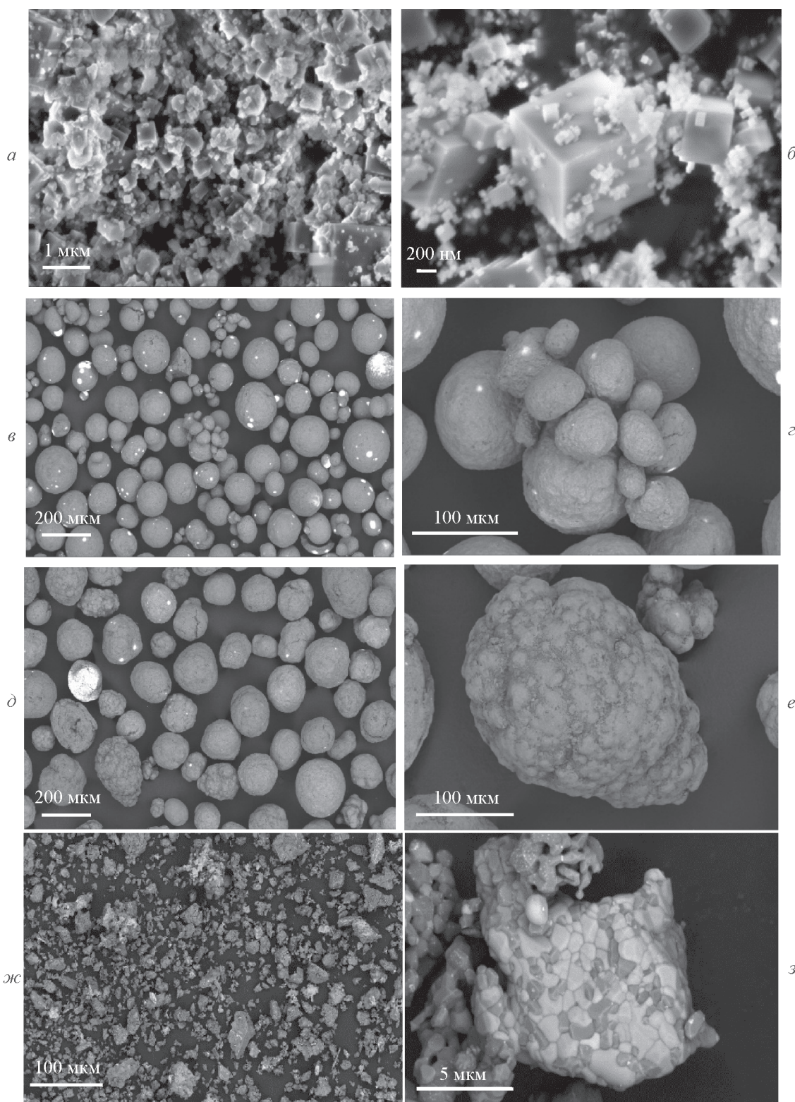
Рис. 2. СЭМ-изображения образцов оксида магния № 1 ( a, б ), 2 ( в, г ), 3 ( д, е ) и 4 ( ж, з ) в обратно-отраженных электронах при различном увеличении.
