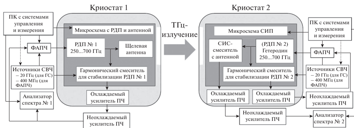
Рис. 4. Схема экспериментальной установки для измерения излучения генератора на основе РДП, расположенного в криостате 1, в открытое пространство с помощью ТГц-спектрометра на основе СИП, расположенного в криостате 2.
