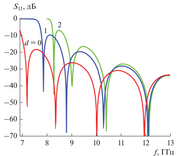
Рис. 9. Коэффициент отражения в структуре на рис. 8 для величин зазора d = 0, 1, 2 .
