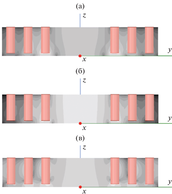
Рис. 6. Распределения амплитуды поля основной волны в поперечном сечении трехрядного волновода с параметрами P = 6, D = 3, h = 10 для зазора d = 1 на разных частотах: а – 7.570 ГГц (критическая частота, фазовый сдвиг 0^\circ ), б – 10.846 ГГц (фазовый сдвиг 60^\circ ), в – 17.755 ГГц (фазовый сдвиг 120^\circ ).
