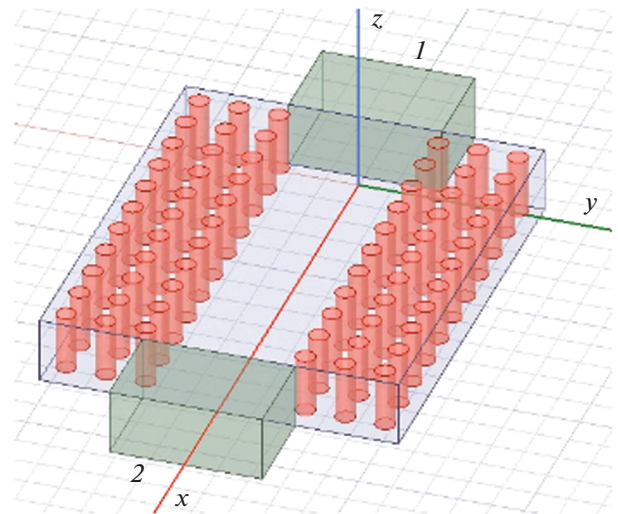
Рис. 8. Модель для расчета матрицы рассеяния секции трехрядного ЕВГ-волновода, состыкованного с двумя прямоугольными металлическими волноводами; 1, 2 – номера портов.
