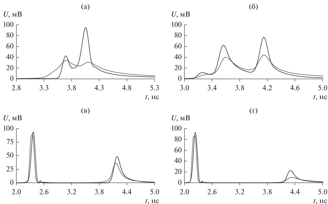
Рис. 4. Формы напряжений на выходе трехпроводного микрополоскового МФ при оптимизации ЭС (а) и ГА (б) и двухпроводного МФ с лицевой связью при оптимизации ЭС (в) и ГА (г), полученные в результате квазистатического (пунктирная) и электродинамического (сплошная) анализа.
