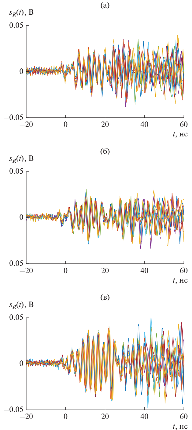
Рис. 5. Реализации 10 хаотических радиоимпульсов на выходе антенны АЗ, совмещенные по времени их начала, при передаче на антенну сигнала от каждой пары G1–А1 (а) и G2–А2 (б) и при передаче сигнала одновременно от G1–А1 и G2–А2 (в).
