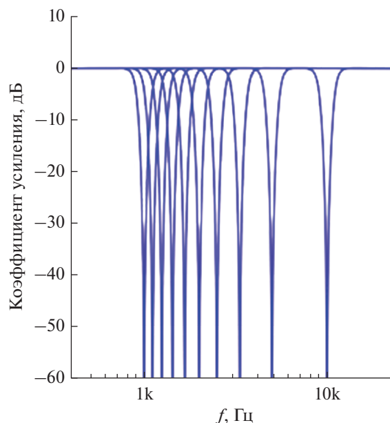
Рис. 8. Перестройка частоты режекции фильтра без изменения ширины заграждения.
