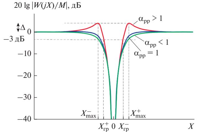
Рис. 5. Графическое определение параметров АЧХ при разных коэффициентах передачи α pp .
