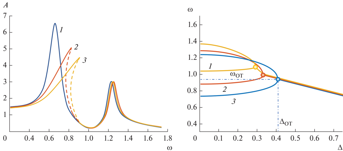
Рис. 1. Семейство амплитудно-частотных характеристик двух связанных осцилляторов Дуффинга (а) и зависимости действительных частот нормальных частот от величины вносимых потерь (б) для трех значений коэффициента нелинейности: \beta = 0 (1), 1 (2) и 3 (3); штрихпунктирной линией обозначены неустойчивые области резонансной кривой.
