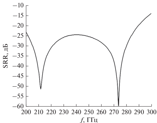
Рис. 7. Зависимость уровня разделения полос SRR от частоты, построенная на основе баланса одного волноводного гибридного делителя.
