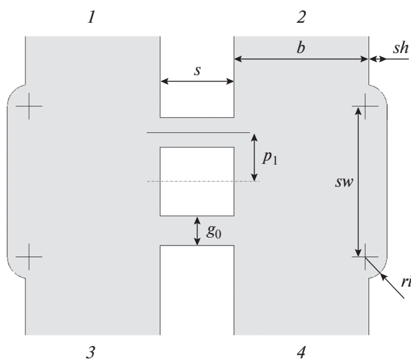
Рис. 8. Волноводный направленный ответвитель: 1–4 – порты, b = 500 , s = 276 , g_0 = 108 , p_1 = 183 , sw = 560 , sh = 67 , ri = 80 . Все размеры даны в мкм.
