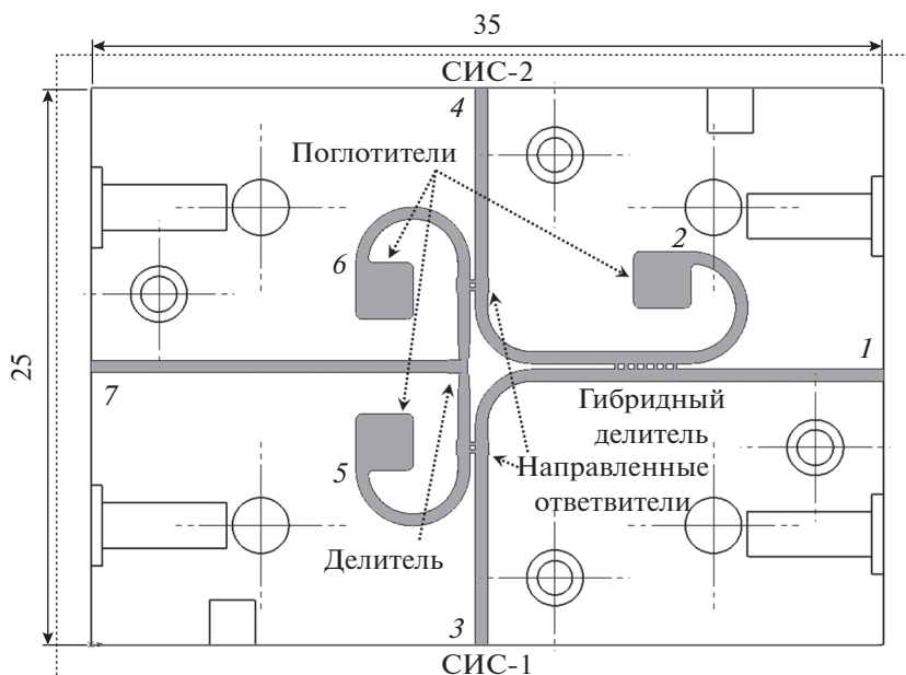
Рис. 2. Волноводный сплит-блок диапазона 211...275 ГГц с разделением боковых полос на основе пары СИС-смесителей: серым выделена волноводная структура, 1–7 – номера портов, СИС-1 и СИС-2 – выходы, на которых будут размещаться волноводные камеры с СИС-смесителями).
