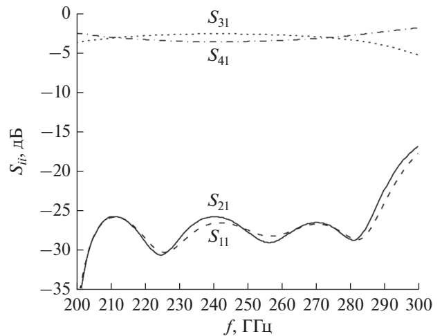
Рис. 4. S -параметры гибридного делителя.
