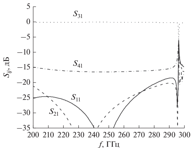
Рис. 9. Частотные характеристики волноводного ответвителя.
