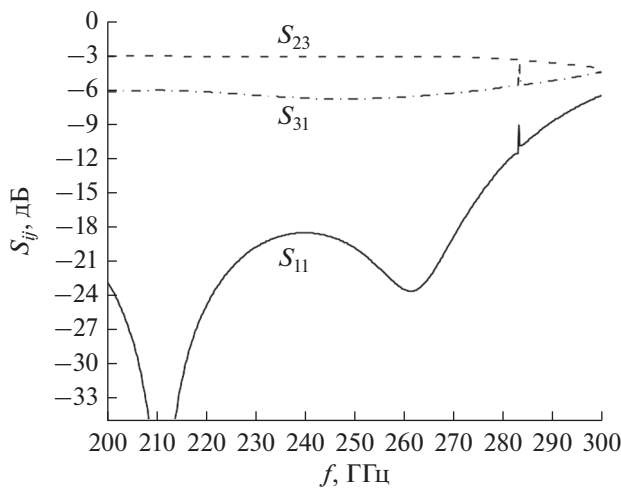
Рис. 11. Частотные характеристики делителя мощности опорного генератора.
