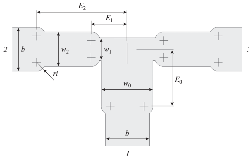
Рис. 10. Делитель мощности опорного генератора, b = 500 , w_0 = 587 , w_1 = 259 , w_2 = 394 , E_0 = 649 , E_1 = 415 , E_2 = 1039 , r_i = 80 . Все размеры даны в мкм.
