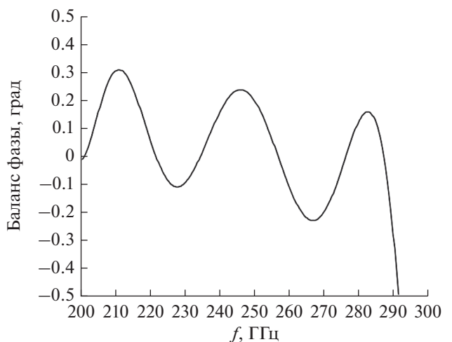
Рис. 6. Фазовый баланс гибридного делителя.
