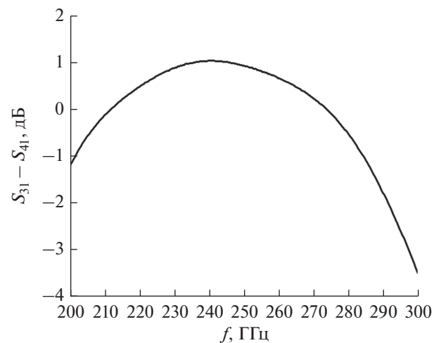
Рис. 5. Амплитудный баланс гибридного делителя.
