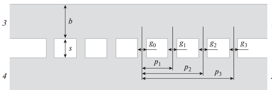
Рис. 3. Схема волноводного гибридного делителя: 1...4 – порты гибрида; g_0 = 124 , g_1 = 124 , g_2 = 116 , g_3 = 108 – ширины щелей; p_1 = 428 , p_2 = 856 , p_3 = 1284 , обозначают положение щелей относительно середины центральной щели g_0 ; s = 290 – расстояние между волноводами гибрида; b = 500 – высота волновода. Все размеры – приведены в мкм.
