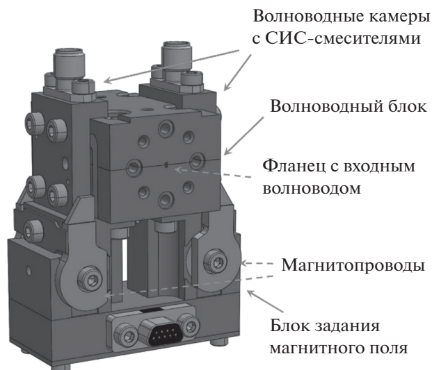
Рис. 1. Приемник диапазона 211...275 ГГц с разделением боковых полос на основе пары СИС-смесителей.
