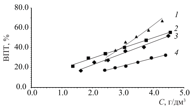
Рис. 6. Зависимость выхода по току (ВПТ) от концентрации оксалат-ионов в растворе 10 г/дм³ \text{NaNO}_3 с pH 10.0 (1) и в том же растворе, дополнительно содержащем хлорид (2), сульфат (3) и борат-ионы (4). I = 0.8 А, U = 2.9 В.
