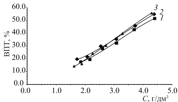
Рис. 5. Зависимость выхода по току (ВПТ) от концентрации оксалат-ионов в растворах с различной концентрацией \text{NaNO}_3 , г/дм³: 1 – 1.0, 2 – 10, 3 – 150. pH 10.0. I = 0.8 А, U = 2.9 В.
