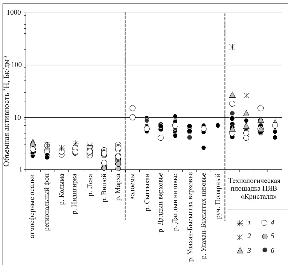
Рис. 4. Объемная активность трития ( \text{Бк/дм}^3 ) в поверхностных стоках технологической площадки ПЯВ «Кристалл» и в речной воде прилегающей территории в разные годы. Условные обозначения: 1 – 2000 г.; 2 – 2002 г.; 3 – 2008 г.; 4 – 2012–2014 гг.; 5 – 2016 г.; 6 – 2018–2020 гг. Точки отбора проб см. рис. 1–3. Течение р. Улахан-Бысытта от объекта «Кристалл» до устья условно принято за ее низовье, а выше – за ее верховье. Течение р. Далдын выше устья р. Улахан-Бысытта условно принято за ее верховье, ниже – за ее низовье. Для сравнения приведены данные по активности трития в стоках технологической площадки в 2002 г. [2], региональная фоновая активность трития в атмосферных осадках и в речной воде [26–33], активность трития в рр. Колыма, Индигирка, Лена [26, 30], в рр. Вилюй, Марха [34].
