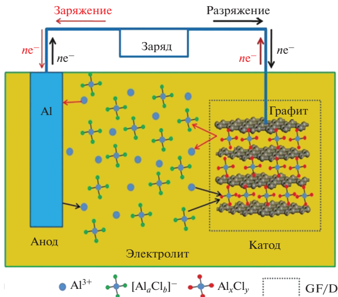
Рис. 1. Принцип работы алюминиев-ионного источника тока с 1-этил-3-метилимидазолхлоридом в качестве электролита и углеродным катодом [9].
