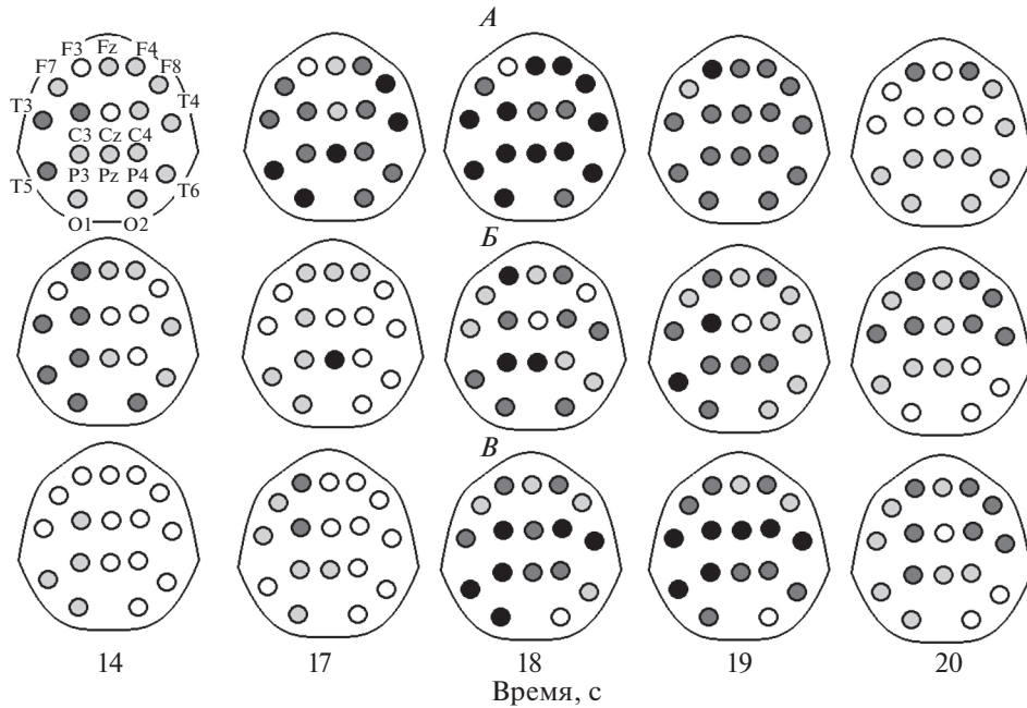
Рис. 5. Карты-схемы статистически значимых изменений в мощностных характеристиках биоэлектрических колебаний разных частотных диапазонов перед пробуждением. По вертикали: А, Б, В – дельта-, медленные альфа-, быстрые альфа-колебания соответственно; по горизонтали: секундные интервалы исследуемого отрезка ЭЭГ (20 с); белые, светло-серые, темно-серые и черные круги – отсутствие значимости, p < 0.05 , p < 0.01 и p < 0.001 соответственно. Значимости приведены по отношению к спектральным характеристикам ЭЭГ на первой секунде исследуемого отрезка записи. На карте-схеме в левом верхнем рисунка показаны названия отведений, для которых проводился статистический анализ.
