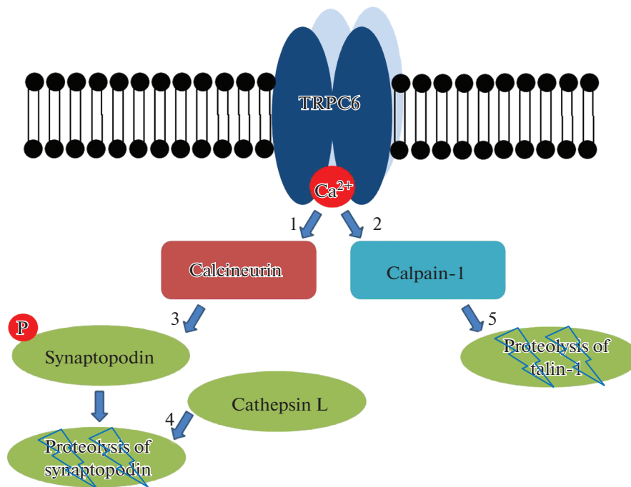
Рис. 3. Схема \text{Ca}^{2+} -зависимой активации кальцинейрина и кальпаина.
