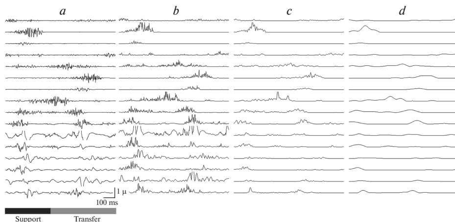
Рис. 3. Образцы ЭМГ скелетных мышц туловища, верхних и нижних конечностей при выполнении локомоций умеренной интенсивности в различных периодах бегового шага. (а) – интерференционная, (б) – выпрямленная, (с) – фильтрованная полосовым фильтром 25–450 Гц, (д) – фильтрованная полосовым фильтром 25–450 Гц + повторная фильтрация ФНЧ 20 Гц.
