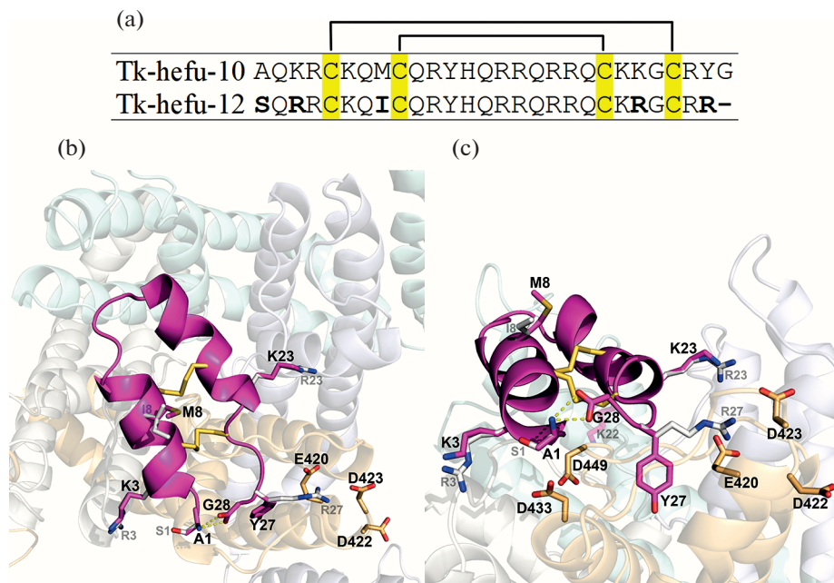
Рис. 1. Аминокислотные последовательности исследуемых пептидов и модель комплекса Тк-hefu-10 с каналом K_v1.3 . (a) – Сравнение аминокислотных последовательностей Тк-hefu-10 и 12. Остатки цистеина выделены желтым, показано расположение дисульфидных связей. (b) – Модель комплекса Тк-hefu-10– K_v1.3 после 200 нс МД в гидратированном липидном бислое. Вид внешнего вестибюля поры канала. (c) – Вид со стороны клеточной мембраны. Субъединицы канала (показаны полупрозрачно на заднем плане) и пептид (показан розовым цветом) представлены в виде ленточных моделей. Затыкающий пору канала остаток K22 (полупрозрачный на панели c), некоторые остатки пептида Тк-hefu-10, выбранные для замены/делеции, возможное положение боковой цепи остатков S1, R3, I8, R23 и R27 (показаны белым цветом) и дисульфидные мостики в пептиде Тк-hefu-12, а также некоторые отрицательно заряженные остатки канала показаны стержневыми моделями. Желтыми пунктирными линиями обозначены полярные контакты между N- и C-концевыми остатками пептида. Визуализация выполнена с помощью программы РuMOL.
