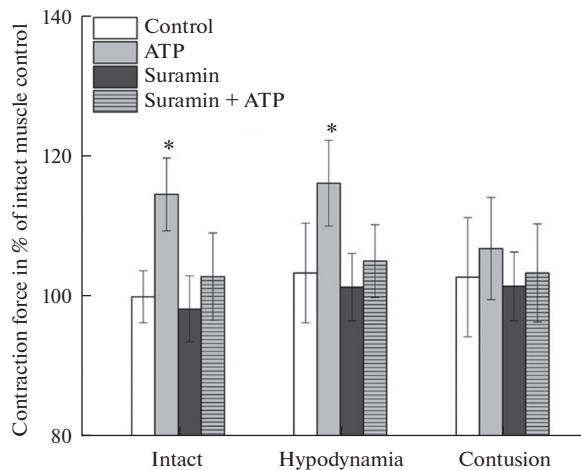
Рис. 3. Зависимость силы сокращений m. diaphragm крыс, вызванных электрической стимуляцией, от экспериментальных условий в контроле и добавлении в среду АТФ (100 мкМ), сурамина (100 мкМ) или их сочетания. n = 7-12 . * p < 0.05 по сравнению с контролем.
