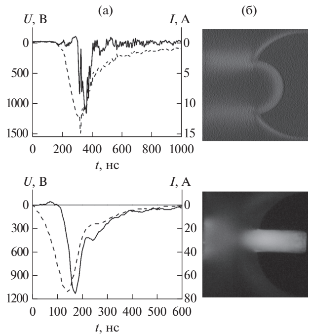
Рис. 2. Осциллограммы (а) напряжения горения (штриховая линия) и разрядного тока (сплошная линия); (б) – пространственное распределение оптического излучения разряда в аргоне ( p = 5 Торр).
