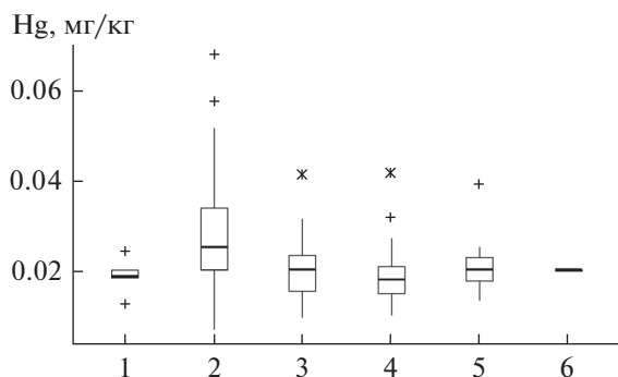
Рис. 1. Содержание ртути в листьях тополя на урбанизированных территориях разных географических регионов Крымского полуострова: 1 – северный, 2 – центральный, 3 – юго-западный, 4 – восточный, 5 – южный, 6 – юго-восточный; * – значимые различия ( p < 0.001 ) по сравнению с центральным регионом, критерий Краскела–Уоллиса.
