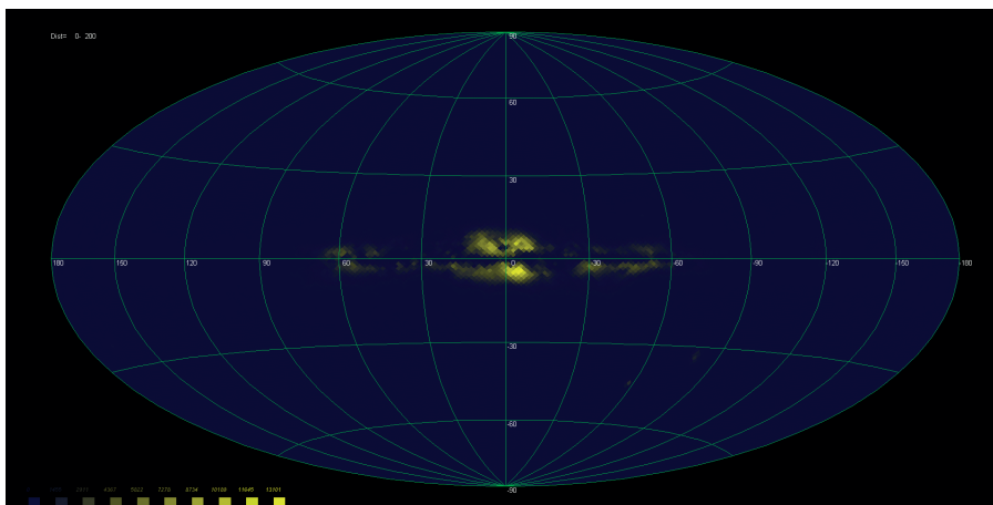
Рис. 8. Распределение Gaia DR3 по небесной сфере для звёзд расстояний (относительная точность параллакса <100\% ) от 0 до 200 пк (максимальная плотность — около 13 000 звёзд на пиксель, 1 пиксель = 0.83 кв. градуса)
