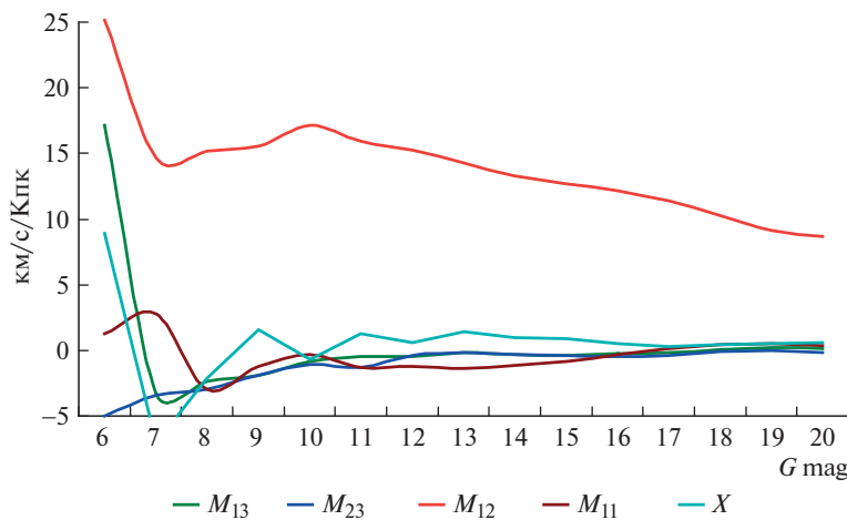
Рис. 21. Зависимость компонент тензора деформации M_{12} , M_{13} , M_{23} , M_{11}^* , X от звёздной величины (км/с/Кпк)
