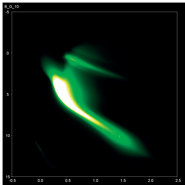
Рис. 14. Диаграмма “показатель цвета V_p-G – абсолютная звёздная величина G ” для звёзд с относительной точностью параллакса лучше 10%
