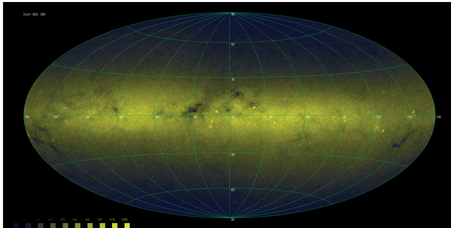
Рис. 10. Распределение Gaia DR3 по небесной сфере для звёзд расстояний (относительная точность параллаксов <10\% ) от 600 до 800 пк (максимальная плотность – около 1200 звёзд на пиксель, 1 пиксель = 0.83 кв. градуса)
