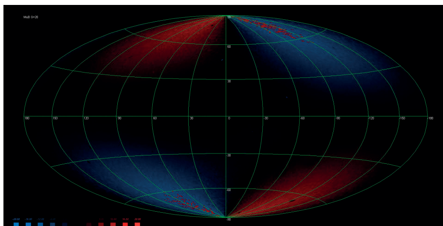
Рис. 18. Поведение собственных движений \mu_b для звёзд G = 20 (от -20 до +20 mas/год)
