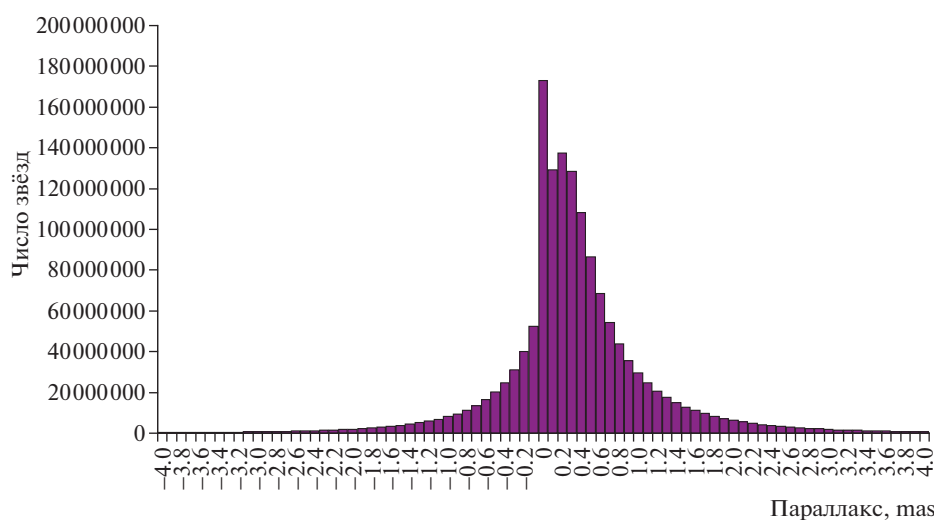
Рис. 3. Распределение звёзд Gaia EDR3 по параллаксам
