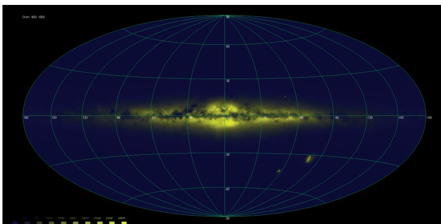
Рис. 9. Распределение Gaia DR3 по небесной сфере для звёзд расстояний (относительная точность параллакса <100\% ) от 800 до 1000 пк (максимальная плотность — около 34 тыс. звёзд на пиксель, 1 пиксель = 0.83 кв. градуса)
