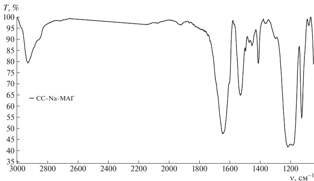
Рис. 2. ИК-спектр сополимера СС-Na-МАГ состава 49 : 51 мол. %.
