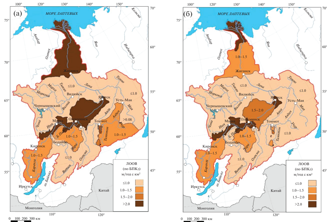
Рис. 3. Среднегодовой модуль стока легкоокисляемых органических веществ (ЛООВ) по БПК 5 в бассейне р. Лены за периоды: а – 2010–2014 гг.; б – 2015–2019 гг.
