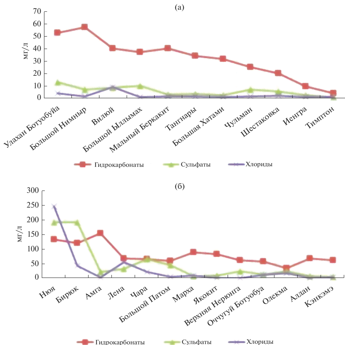
Рис. 2. Среднеголетнее содержание основных анионов в реках бассейна Лены (2010–2019 гг.).
