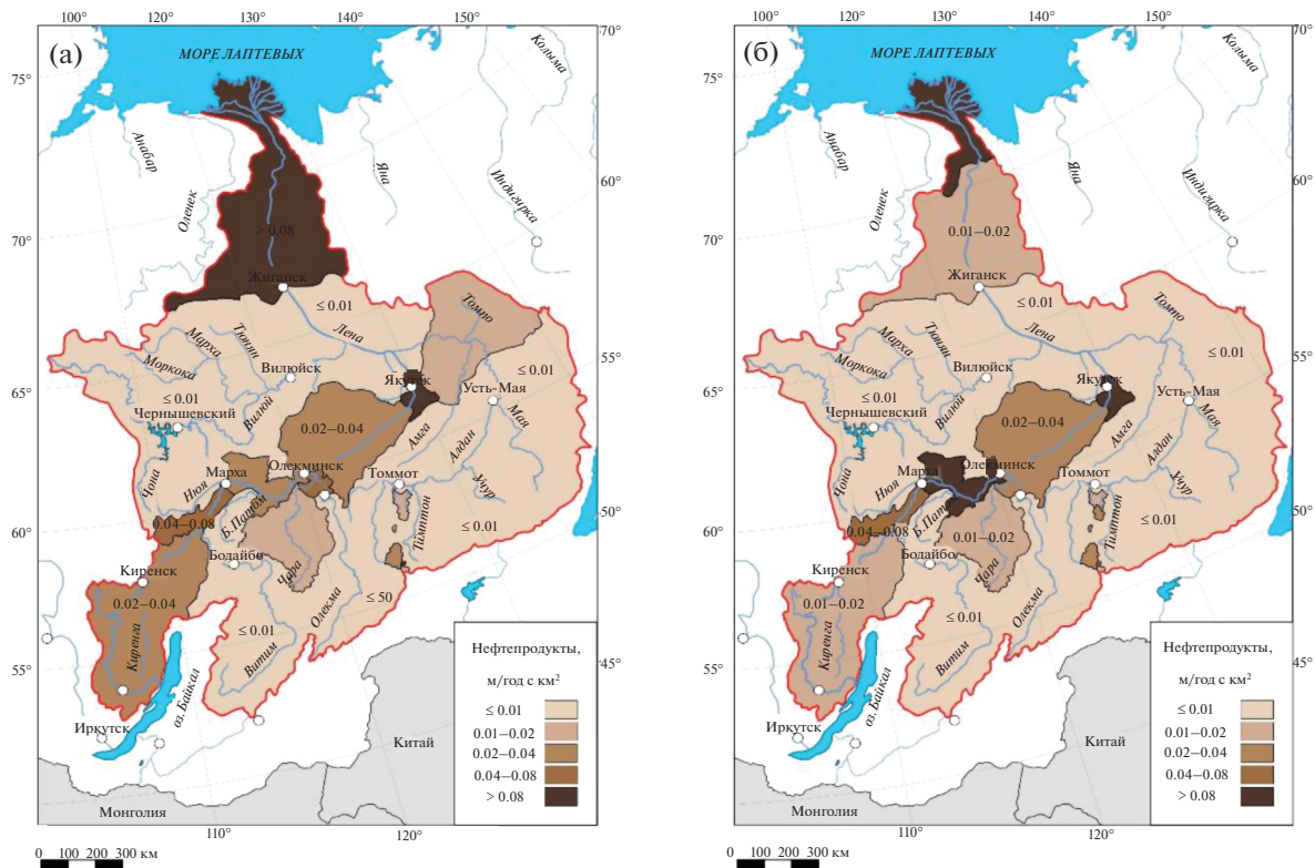
Рис. 5. Среднеголетний модуль стока нефтепродуктов в бассейне р. Лены за периоды: а – 2010–2014 гг.; б – 2015–2019 гг.
