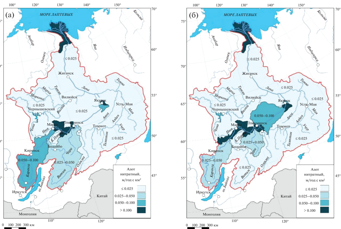
Рис. 6. Среднеголетний модуль стока азота нитратного в бассейне р. Лены за периоды: а – 2010–2014 гг.; б – 2015–2019 гг.
