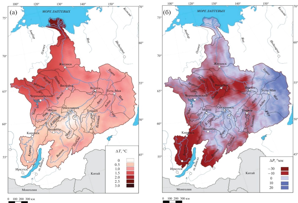
Рис. 1. а – аномалии среднегодовой температуры воздуха T , °С; б – количества осадков P , %, за 2010–2019 гг. относительно 1980–2009 гг.
