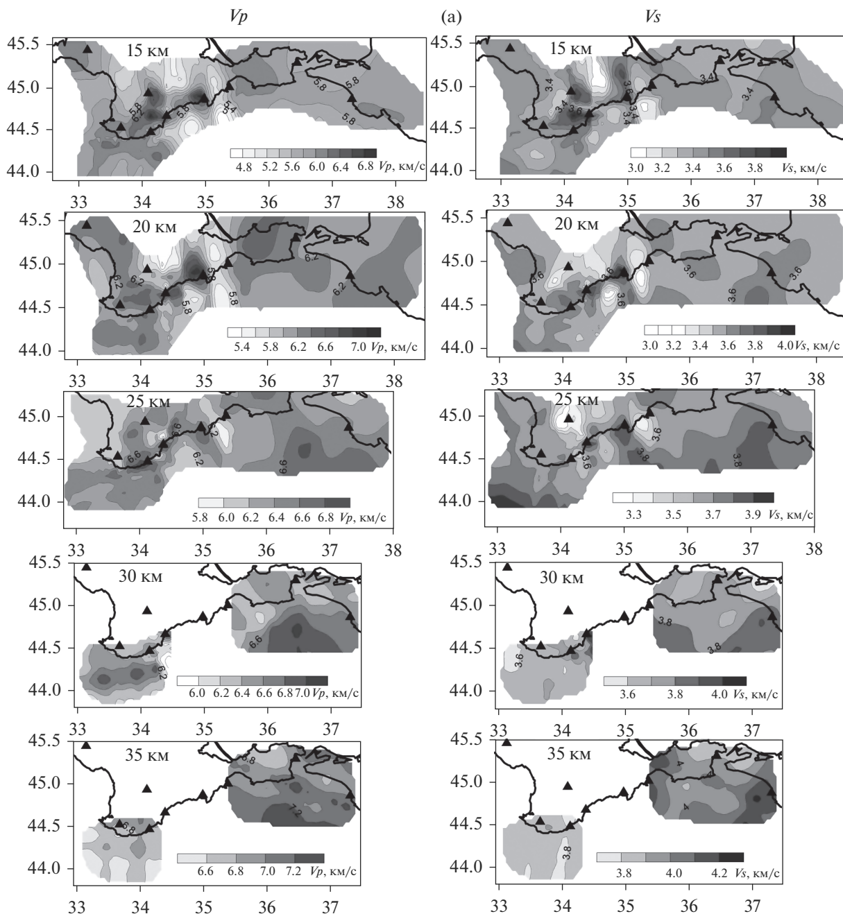
Рис. 4. Распределение скоростей P - и S -волн (а) и соотношения V_p/V_s (б) на глубинах 15–35 км по результатам сейсмо-томографической инверсии времен пробега объемных волн. Черными треугольниками показано положение сейсмических станций.
