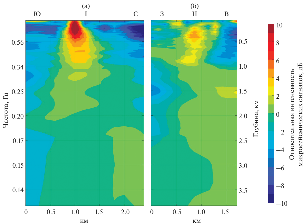
Рис. 4. Распределение спектральных амплитуд микросейсмического шума вдоль профилей, пересекающих вулканическую постройку Джау-Тепе. а – I Юг–Север и б – II Запад–Восток.
