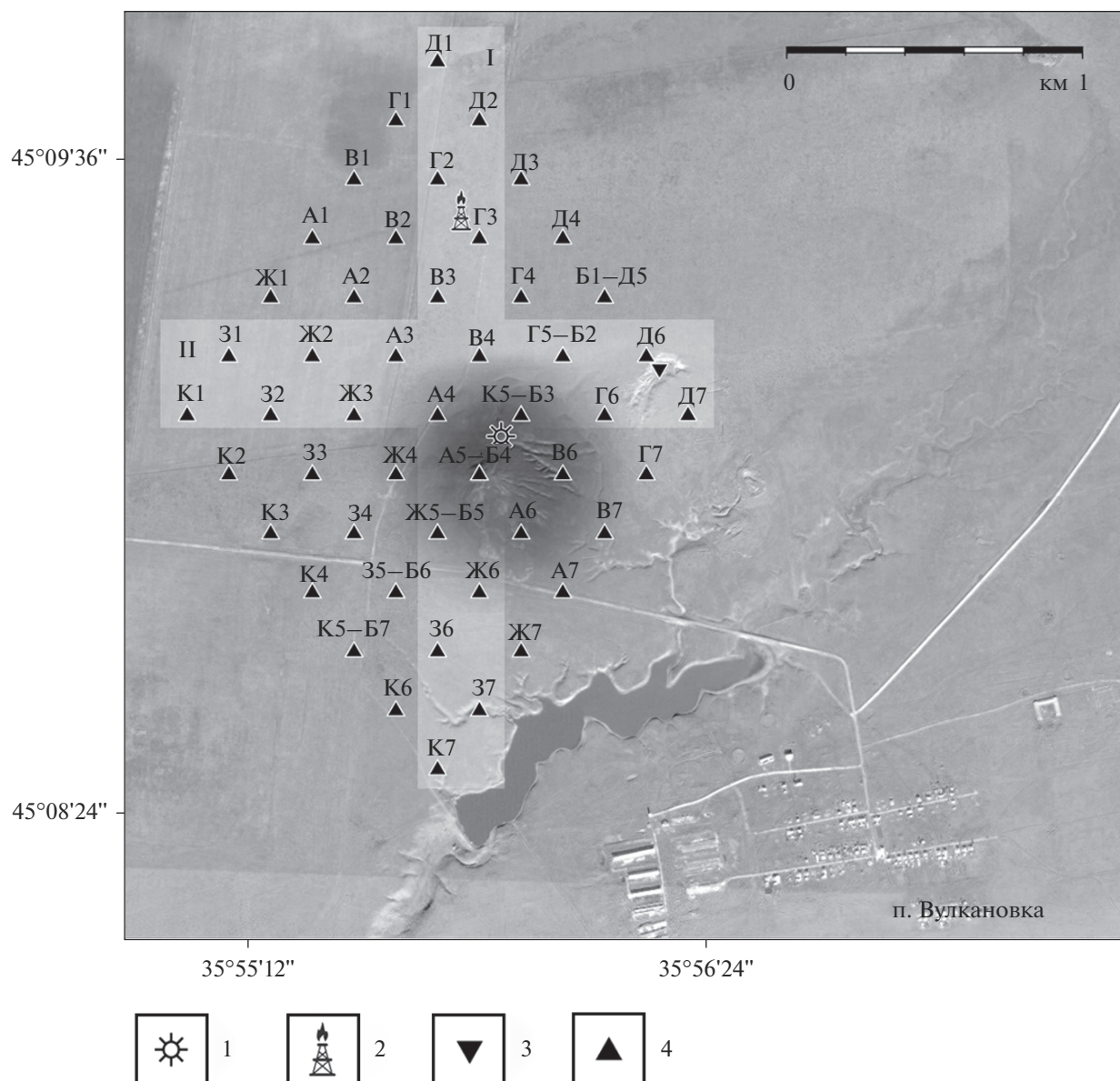
Рис. 1. Грязевой вулкан Джау-Тепе и схема выполнения сейсмических измерений. 1 – новый кратер грязевого вулкана; 2 – разведочная скважина; 3 – вдавленная синклираль; 4 – пункты сейсмических измерений.
