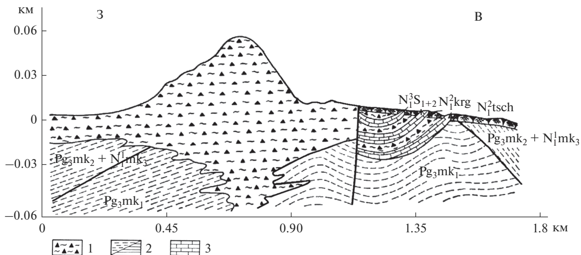
Рис. 6. Геологический разрез сопочного поля Джау-Тепе и выдавленности вдоль профиля П, по [Шнюков и др., 2006] с исправлениями, масштаб осей разный.
