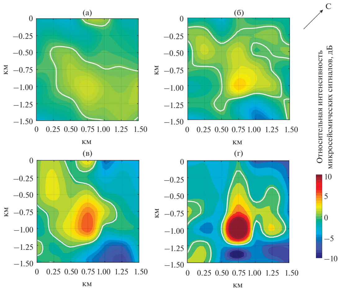
Рис. 7. Горизонтальное распределение относительных амплитуд для различных частотных диапазонов: а – 0.23 Гц, б – 0.33 Гц, в – 0.42 Гц, г – 0.71 Гц.
