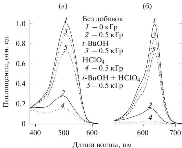
Рис. 2. Полосы оптического поглощения растворов 0.02 \text{ г/дм}^3 E124 (а) и E142 (б) с добавками кислоты и спирта.
