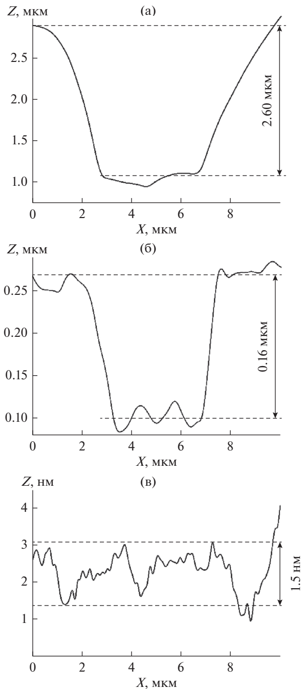
Рис. 6. Профили глубины выемки, образующейся при сканировании участка 4 \times 4 \text{ мкм} в центре изображения с силой прижатия 600 нН, полученные для исходного СВМПЭ ((а) сечение А–А), СВМПЭ обработанного 6 мин в плазме He ((б) сечение В–В), СВМПЭ, обработанного 12 мин в плазме He ((в) сечение А–С) (см. рис. 5), (мощность разряда 50 Вт, поток He 5 \text{ см}^3/\text{мин} при н.у.).
