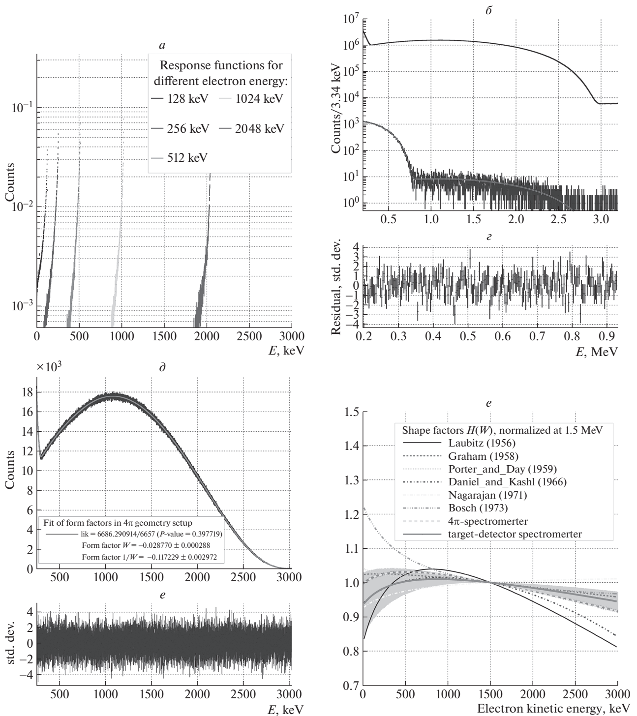
Рис. 2. Для 4 \pi бета-спектрометра функции отклика для электронов, вычисленные методом Монте-Карло ( a ), подгонка перехода 0^- \rightarrow 1^- в ^{144}\text{Pb} ( б ) и разности в терминах стандартных отклонений ( в ), подгонка спектра ^{144}\text{Ce} – ^{144}\text{Pb} ( г ) и разности в терминах стандартных отклонений ( д ), полученные формфакторы в сравнении с результатами предыдущих измерений [7–12] и спектрометра “мишень-детектор” ( е ). Закрашенные области на ( д ) соответствуют статистической неопределенности с одним стандартным отклонением. Можно видеть, что результаты измерений для обоих спектрометров согласуются в пределах статистических неопределенностей.
