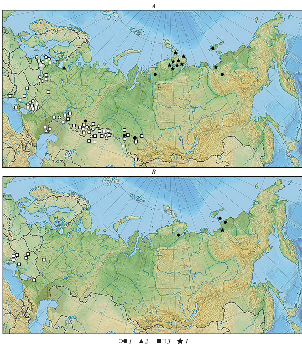
Рис. 2. Места находок костных остатков копытных в SB (А) и SA (В) периодах: 1 – дикая лошадь ( Equus ferus ), 2 – первобытный бизон ( Bison priscus ), 3 – тур ( Bos primigenius ), 4 – овцебык ( Ovibos moschatus ). Закрашенные значки обозначают находки, имеющие абсолютный возраст; значки в виде контуров – находки, датированные на основании радиоуглеродных дат слоя и археологическими методами.
