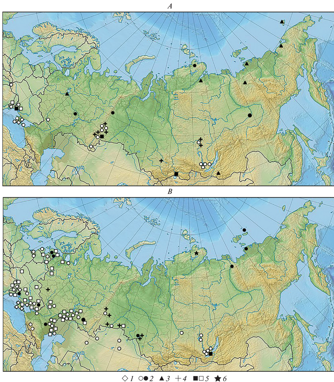
Рис. 1. Места находок костных остатков копытных в РВ–ВО (А) и АТ (В) периодах: 1 – европейский осел ( Equus hydruntinus ), 2 – дикая лошадь ( E. ferus ), 3 – первобытный бизон ( Bison priscus ), 4 – гигантский олень ( Megaloceros giganteus ), 5 – тур ( Bos primigenius ), 6 – овцебык ( Ovibos moschatus ). Закрашенные значки обозначают находки, имеющие абсолютный возраст; значки в виде контуров – находки, датированные на основании радиоуглеродных дат слоя и археологическими методами.
